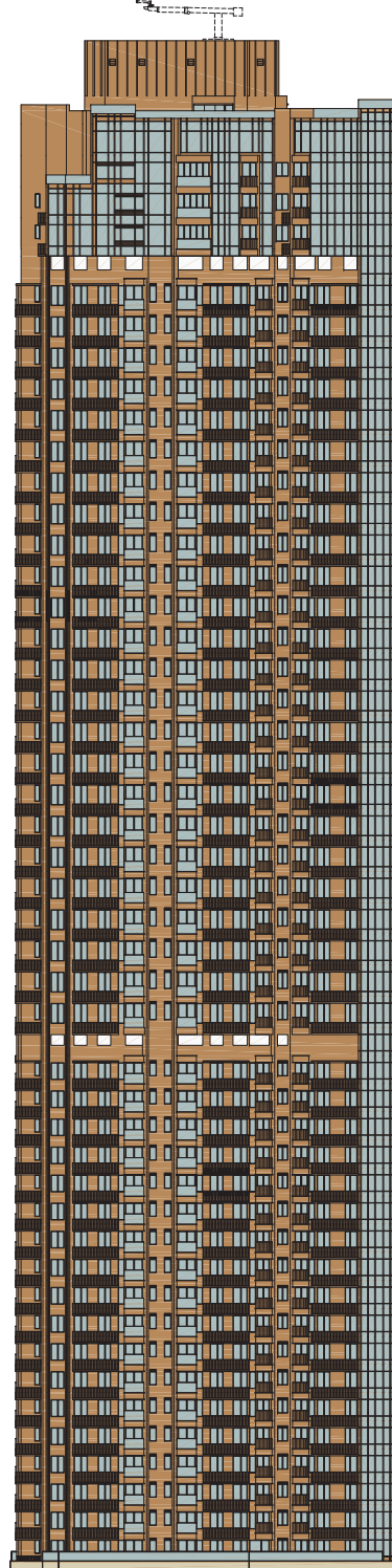
ELEVATION 2 立面圖 2
