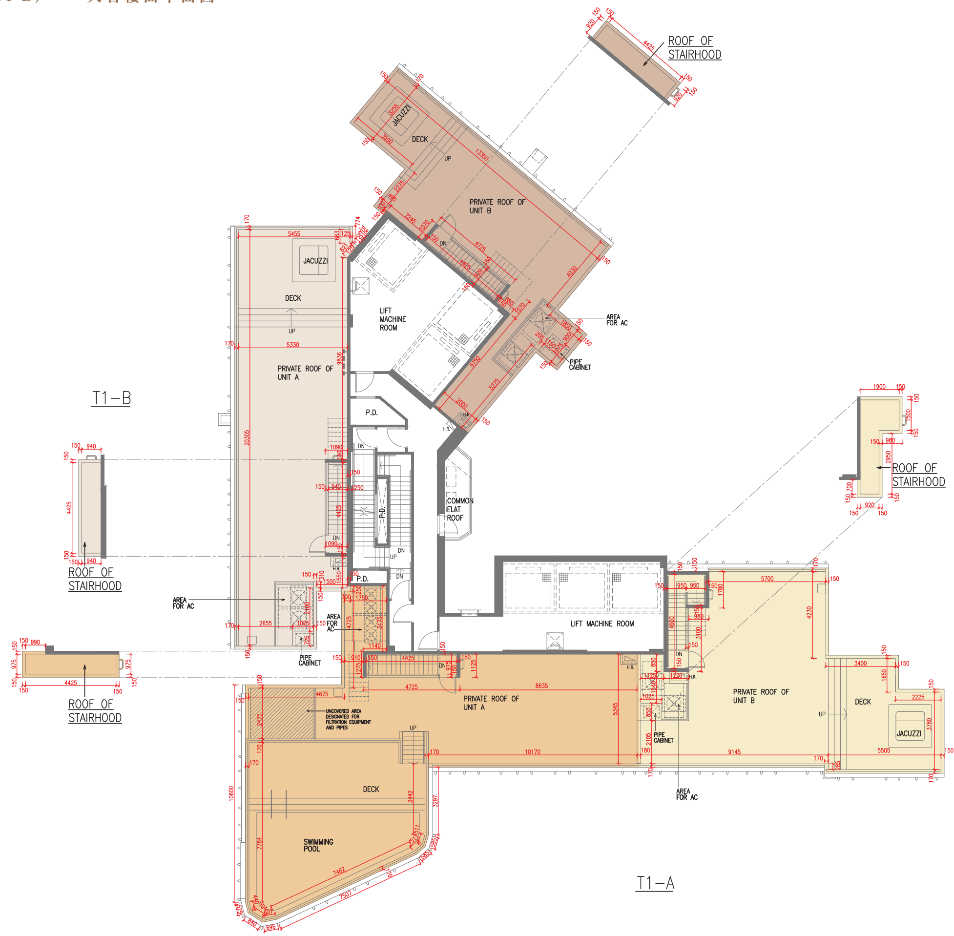
TOWER 1 (T1-A & T1-B) ROOF FLOOR PLAN 第 1 座 (T1-A 及 T1-B) 天台樓面平面圖
