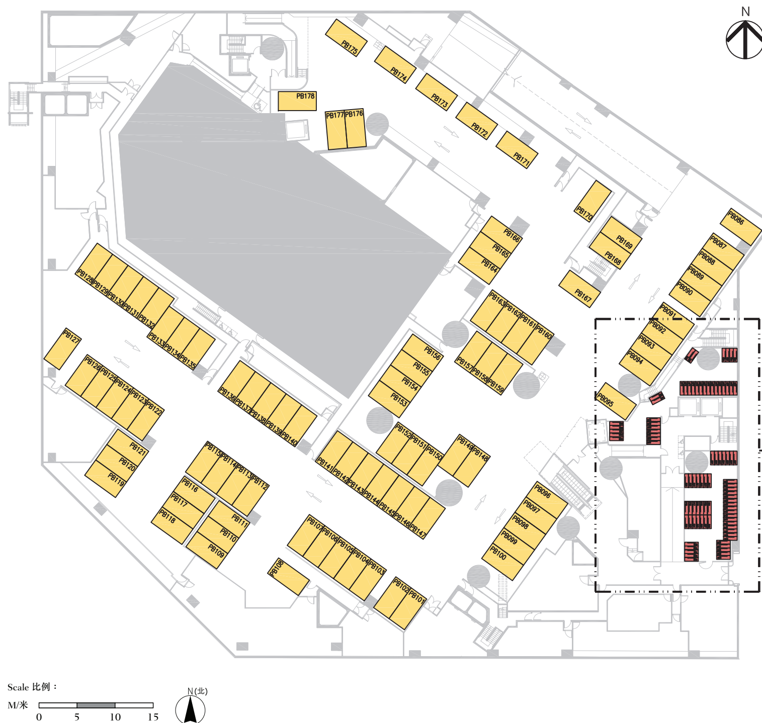
LG2/F CAR PARK FLOOR PLAN 低層地下 2 樓停車場平面圖
